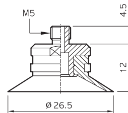
MU25-(N)-M5
