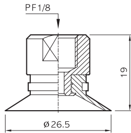
MU25-(N)-18F
