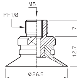
MU25-(N)-18M
