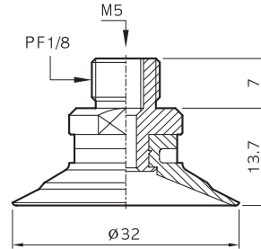
MU30-(N)-18M
