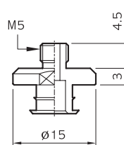
M5-3
