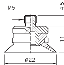
MU20-(N)-M5
