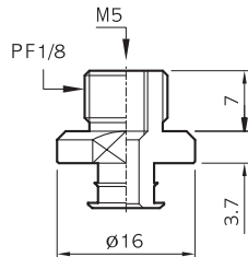
18M-1
