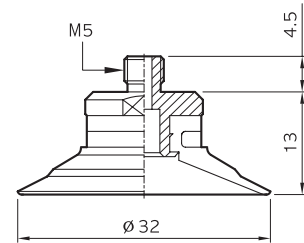
MU30-(N)-M5
