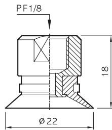
MU20-(N)-18F
