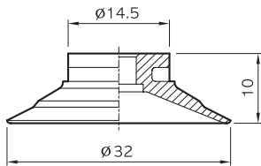
MU30
