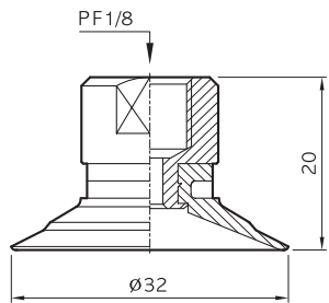
MU30-(N)-18F
